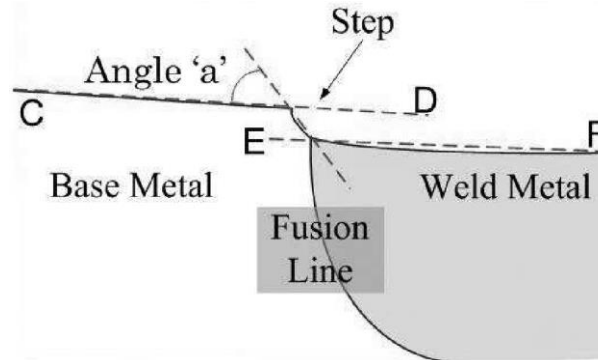
Fig. 2.6.8.3.3.1.1 Calculation of step angle
